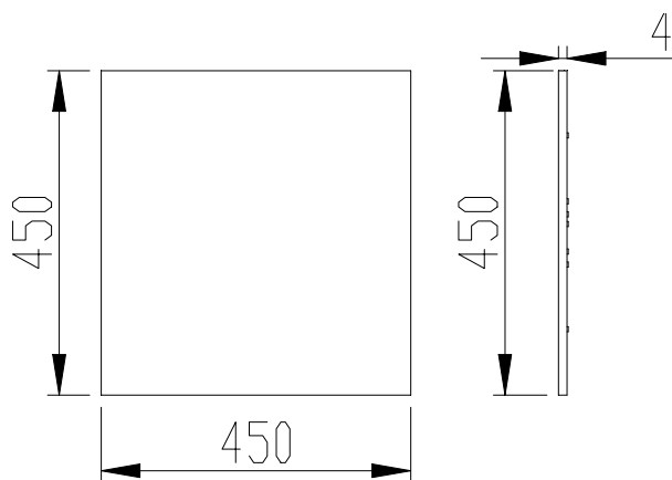
(图4) 铝散热板尺寸图
